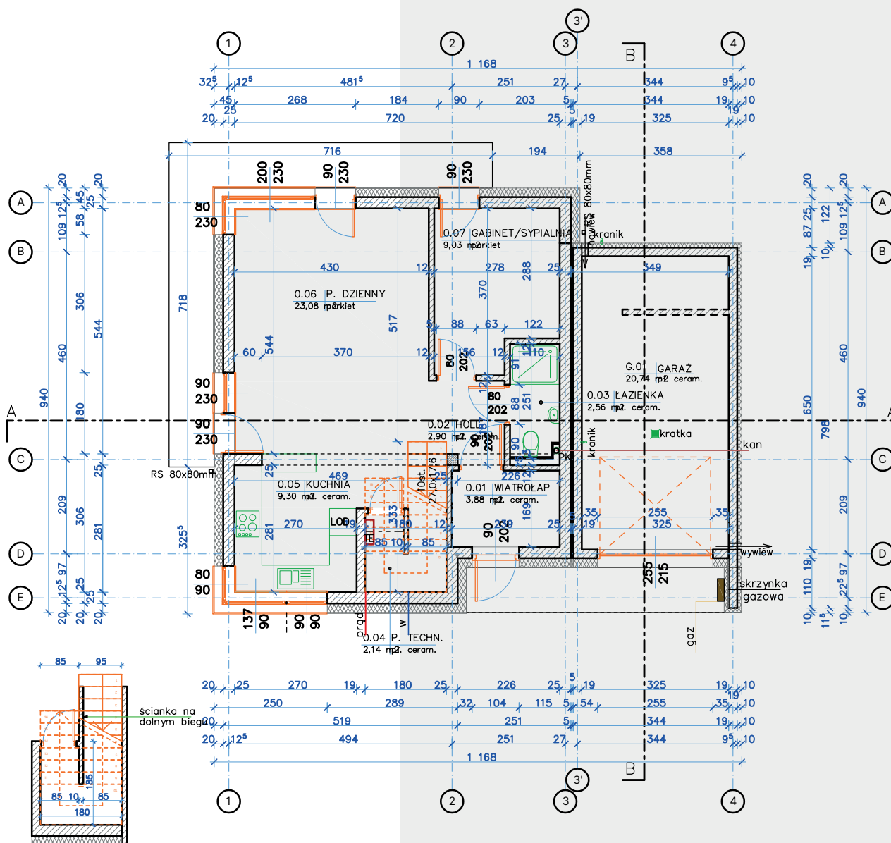
ZESTAWIENIE POWIERZCHNI PARTERU
